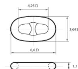
END LINK
