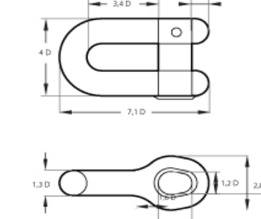
SWIVEL
