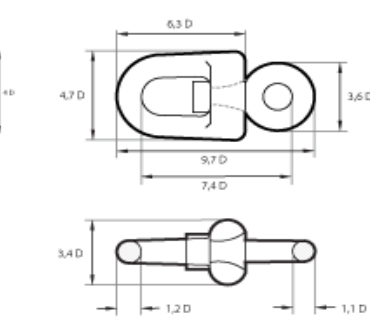
SWIVEL
